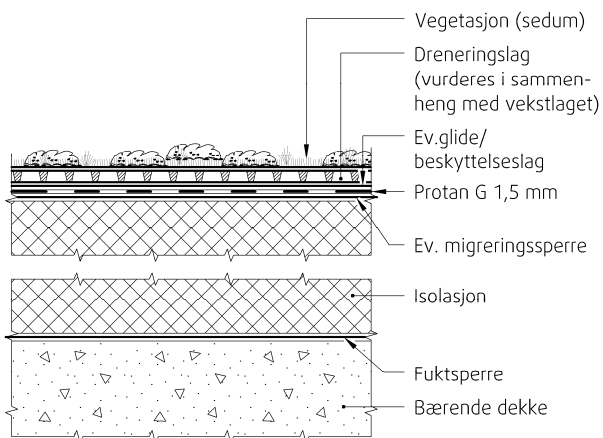
Fig. 7 Protan G brukt som teknisk i ekstensive grønne løsninger
