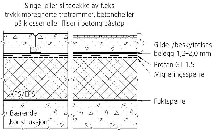
Fig.2 Terrasse, isolert rettventd tak
